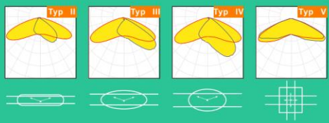
Olika typer av optik
